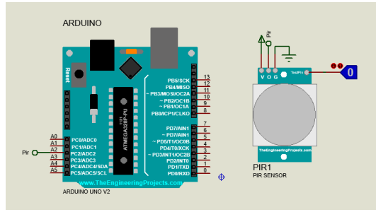
شكل (18) توصيل حساس الحركة بالآردينو
