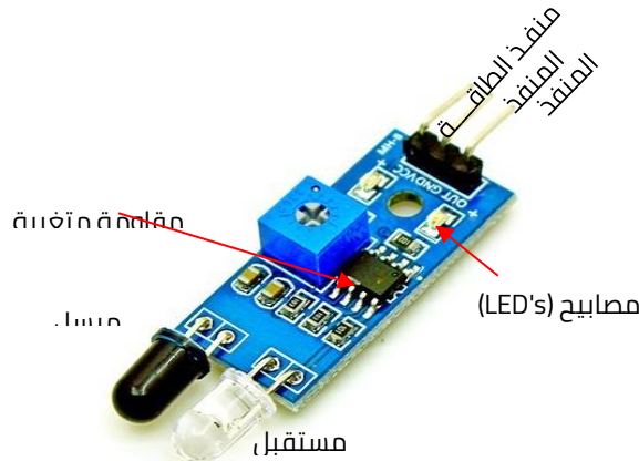
شكل (10) مستشعر العوائق (Infrared Sensor)
