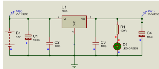
شكل (17) الدائرة الكهربائية المستخدمة لتغذية المنظومة
