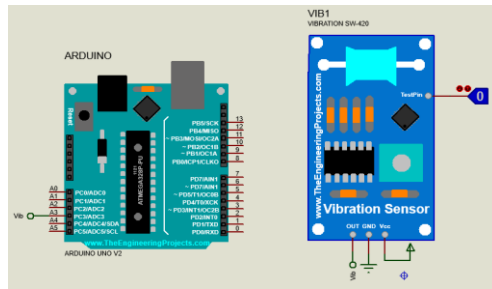
شكل (20) توصيل حساس الاهتزاز
