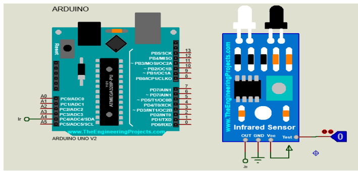
شكل (21) توصيل حساس العوائق
