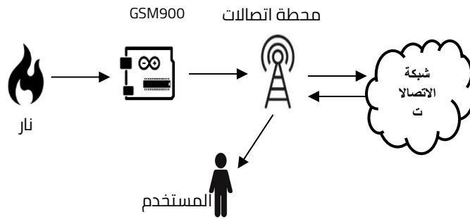
شكل (8) فكرة عمل لوحة (GSM900)
