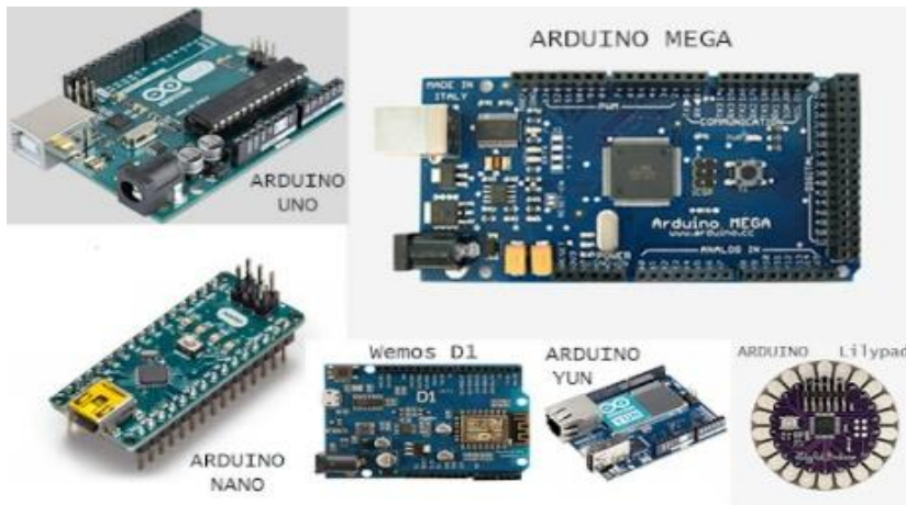
شكل (2) بعض أشكال لوحات الأريدينو
